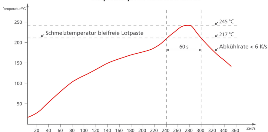
Temperaturprofil Reflowverfahren
